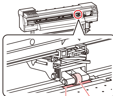
Подающий ролик
