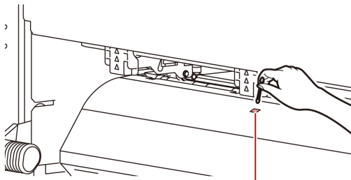
Датчик носителя
